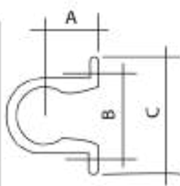
Pipe Clip
